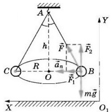
Рис. 2. Расположение сил
