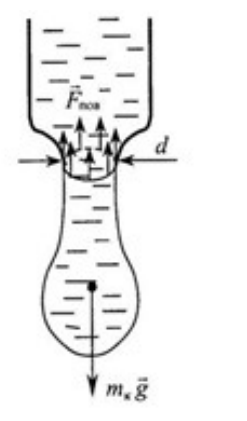
Рис. 2. Метод отрыва капль
