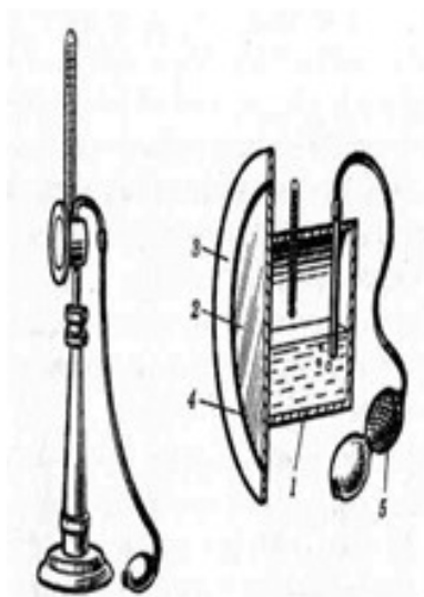
Рис. 2. Гигрометр коденсационный
