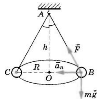
Рис. 1. Конический маятник
