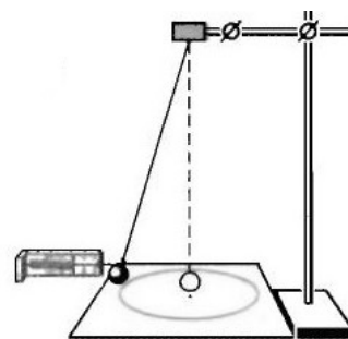
Рис. 3. Определение силы упругости
