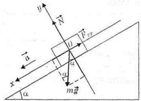
Рис. 1. Тело на наклонной плоскости
